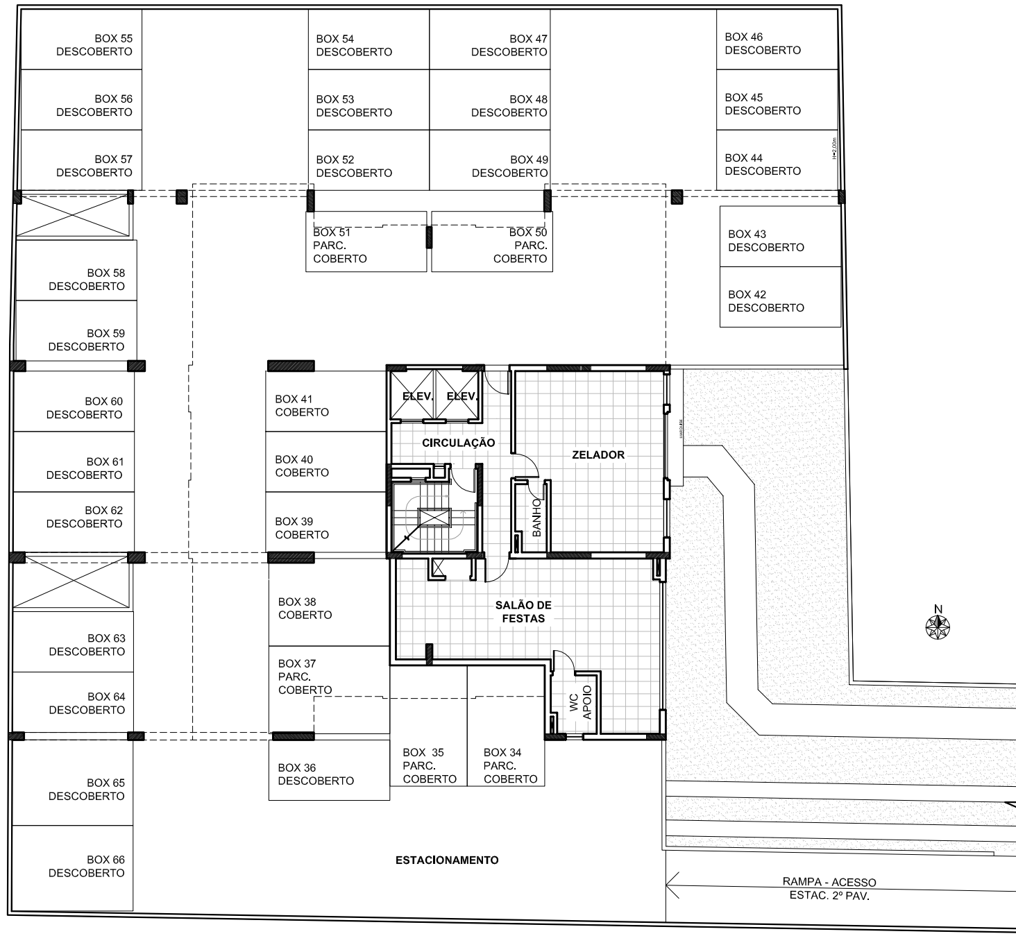
PLANTA BAIXA - 2º PAVIMENTO
