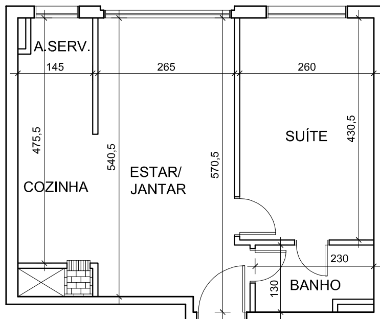
PLANTA BAIXA APARTAMENTO FINAL 05
