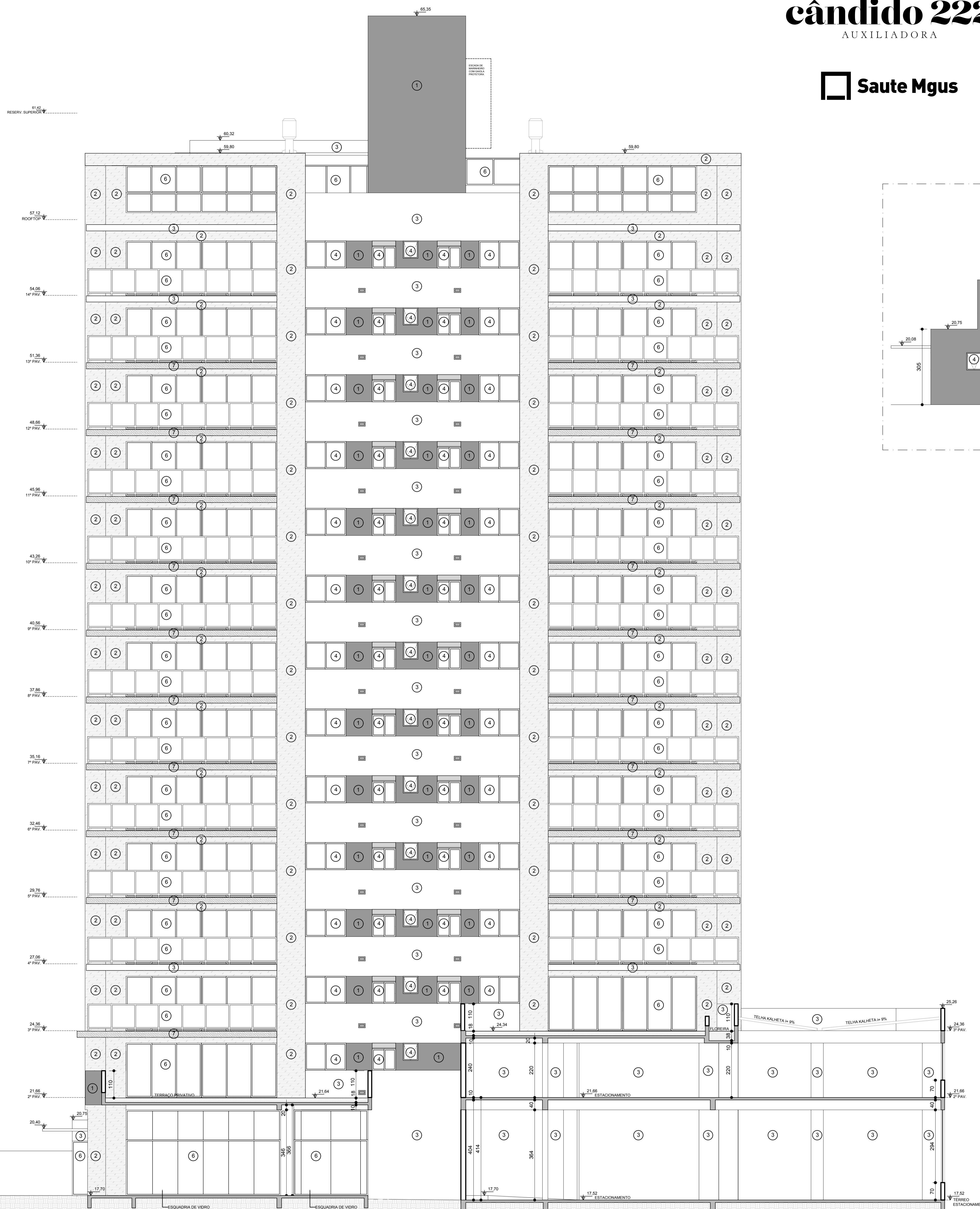
FACHADA SUL ESCALA 1:75
