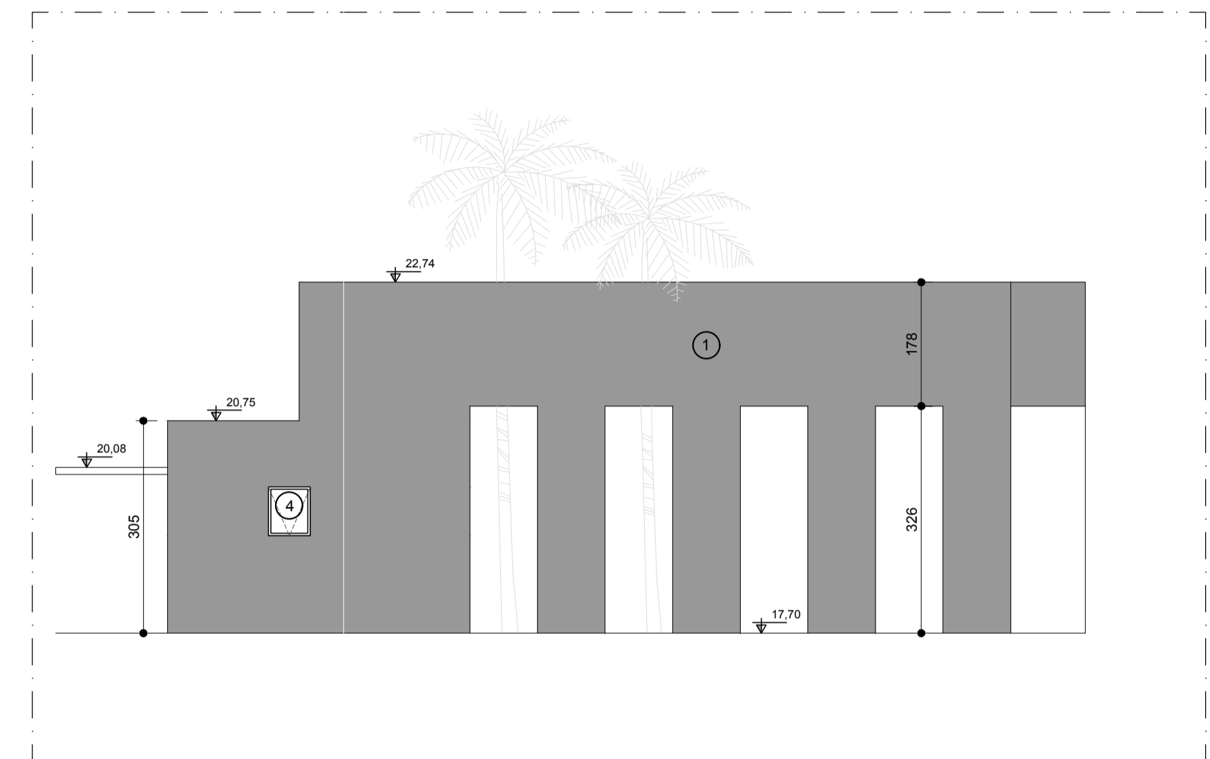
FACHADA SUL - PILOTIS ESCALA 1:75
