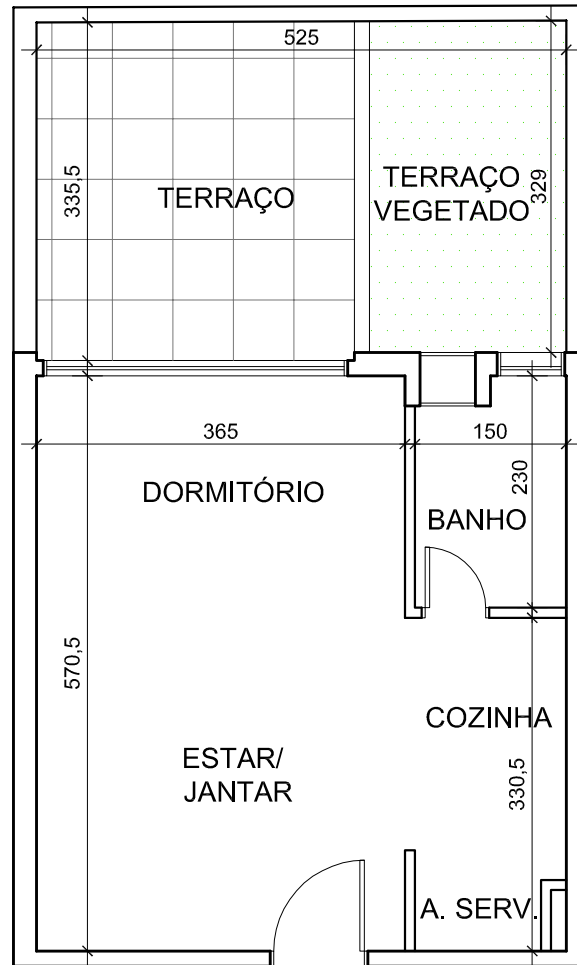
PLANTA BAIXA 3º PAVIMENTO - TORRE FRENTE Av. VENÂNCIO AIRES - APARTAMENTO FINAL 04
