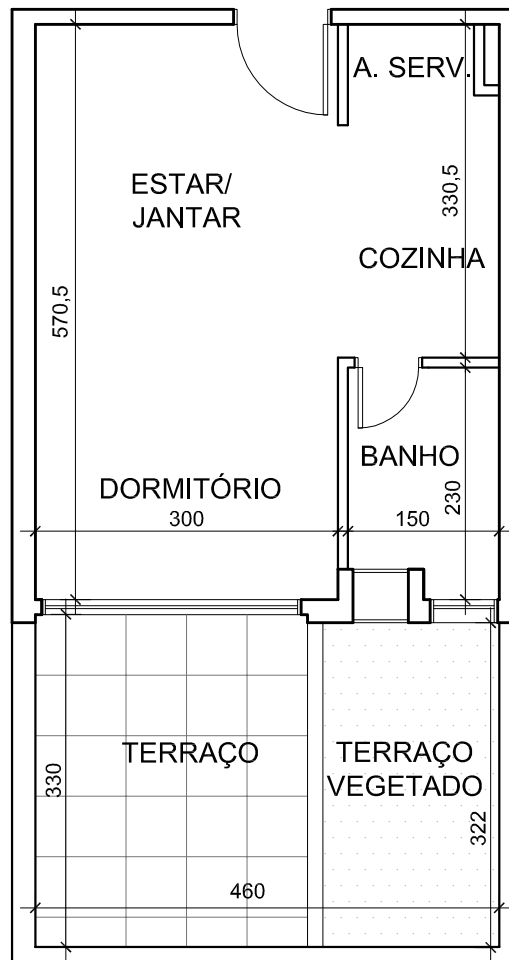
PLANTA BAIXA 3º PAVIMENTO - TORRE FRENTE Av. VENÂNCIO AIRES - APARTAMENTOS FINAIS 09 e 10
