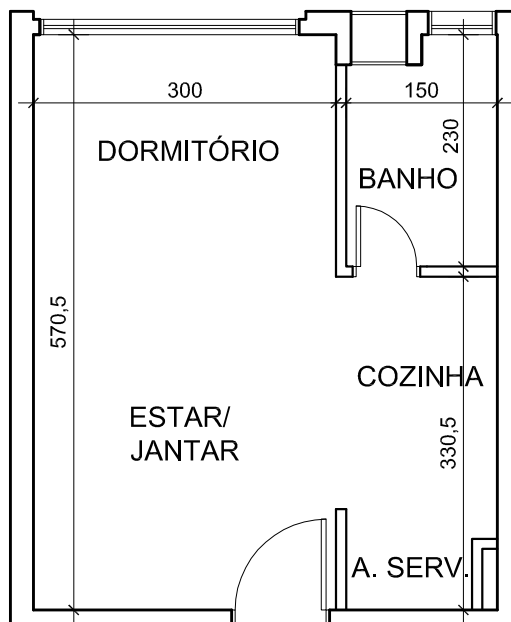
PLANTA BAIXA APARTAMENTOS FINAIS 09 e 10
