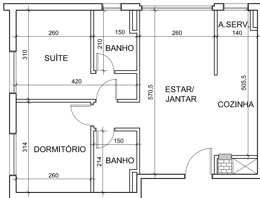
PLANTA BAIXA APARTAMENTOS FINAIS 01, 02, 07 e 08
