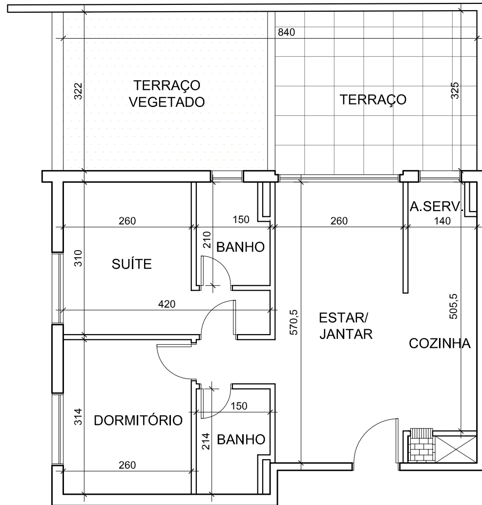
PLANTA BAIXA 3º PAVIMENTO - TORRE FRENTE Av. VENÂNCIO AIRES - APARTAMENTO FINAL 02
