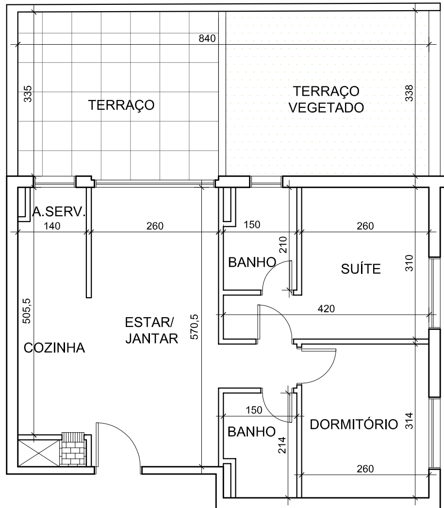
PLANTA BAIXA 3º PAVIMENTO - TORRE FRENTE Av. VENÂNCIO AIRES - APARTAMENTO FINAL 07
