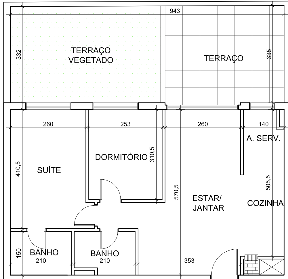
PLANTA BAIXA 3º PAVIMENTO - TORRE FRENTE Av. VENÂNCIO AIRES - APARTAMENTO FINAL 06
