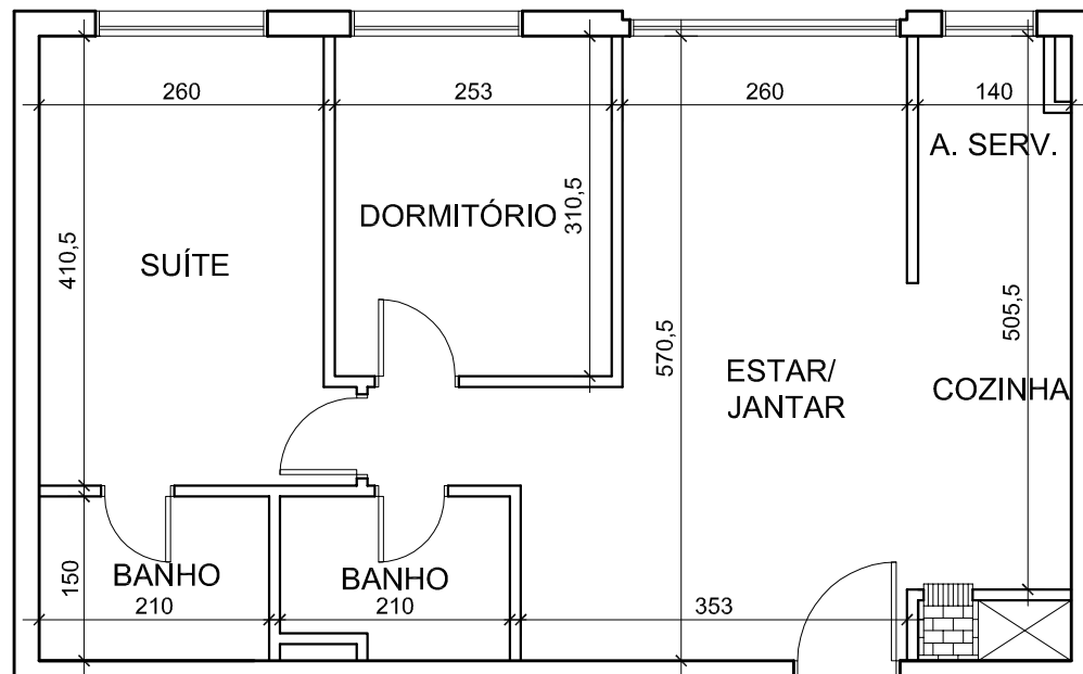
PLANTA BAIXA APARTAMENTO FINAL 06
