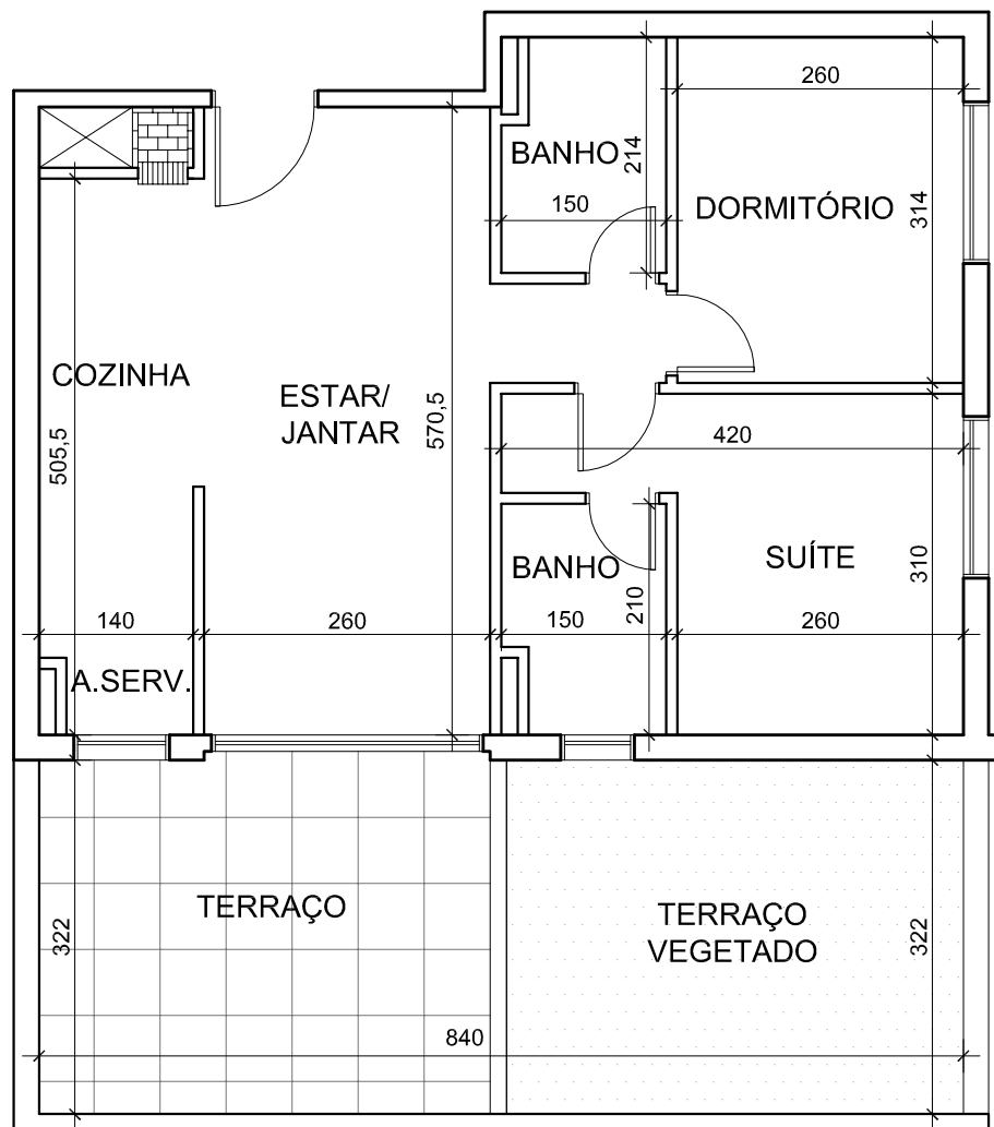
PLANTA BAIXA 3º PAVIMENTO - TORRE FRENTE Av. VENÂNCIO AIRES - APARTAMENTO FINAL 08
